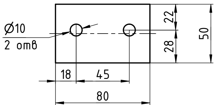
Деталь поз. 3
