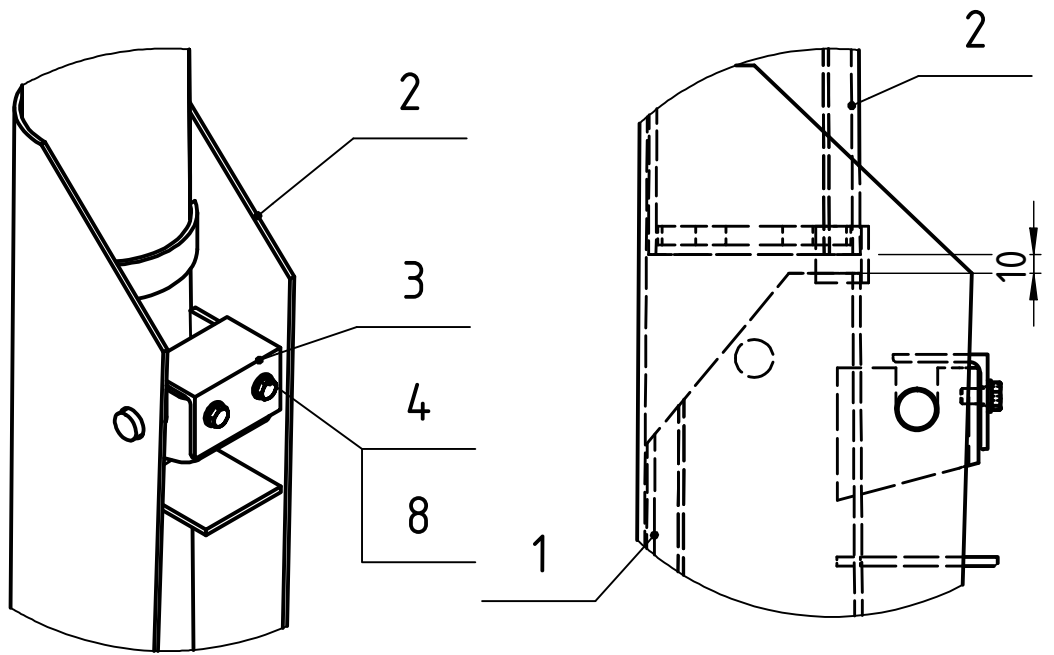
Деталь поз. 3
