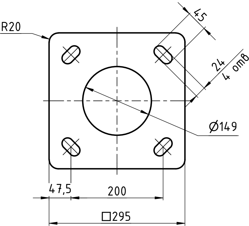
Деталь поз.2
