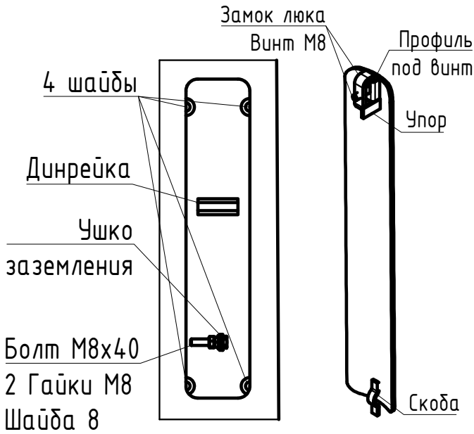
Деталь поз.2
