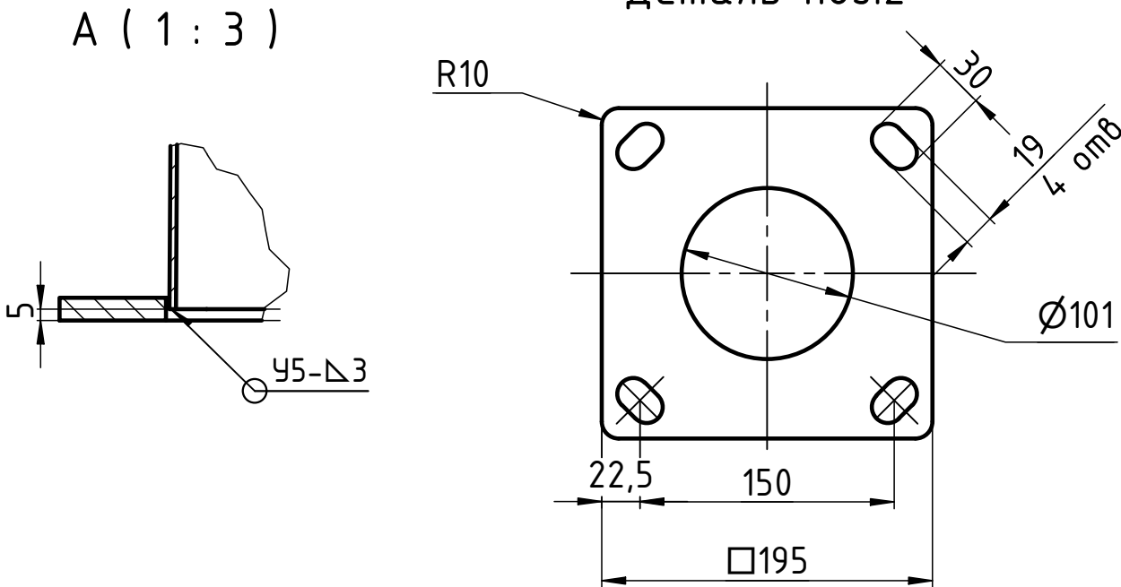
Деталь поз.2
