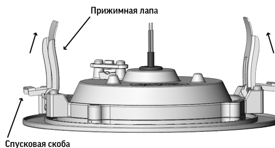
Спусковая скоба
