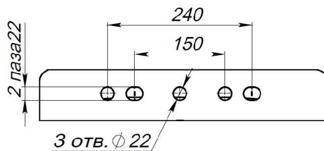
Монтажные отверстия
