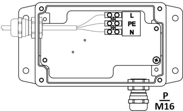
Вводная коробка
