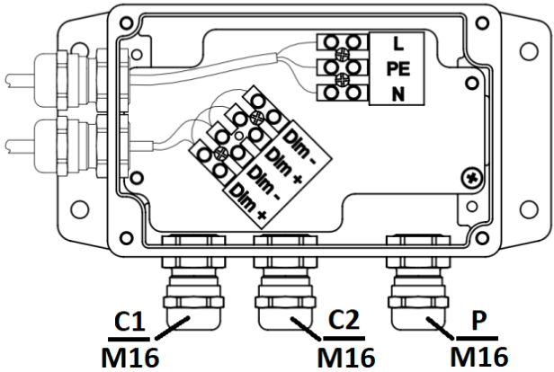
Вводная коробка
