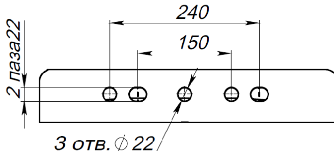
Монтажные отверстия
