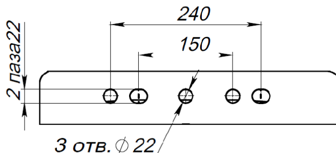
Монтажные отверстия
