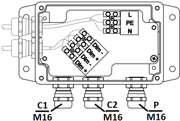
Вводная коробка
