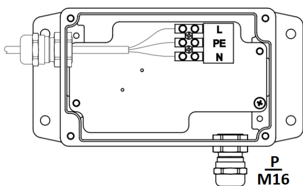
Вводная коробка
