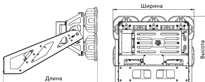
Габаритные размеры прожектора
