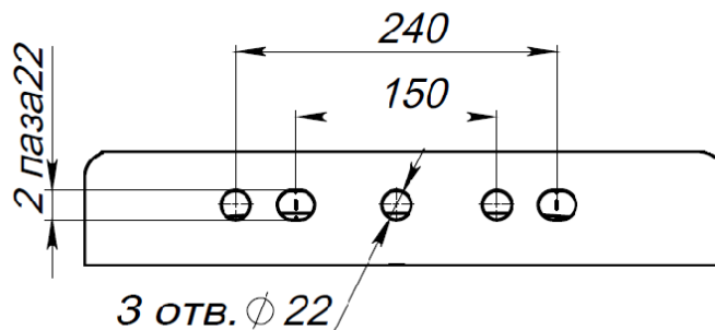
Монтажные отверстия
