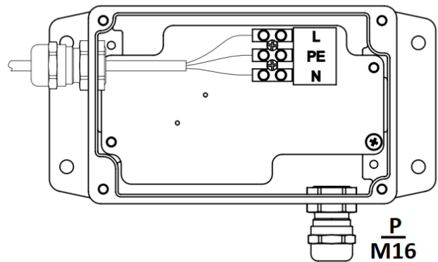
Вводная коробка
