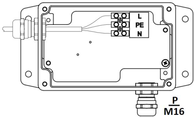
Вводная коробка
