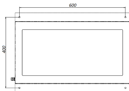
Установочные размеры
