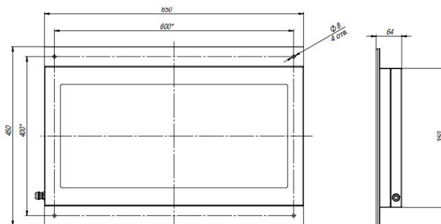
Габаритные размеры
