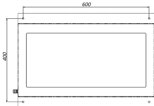
Установочные размеры
