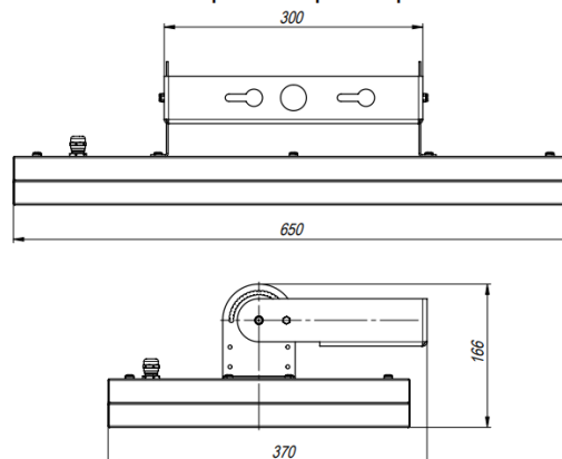
Габаритные размеры
