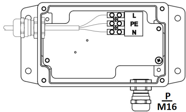
Вводная коробка
