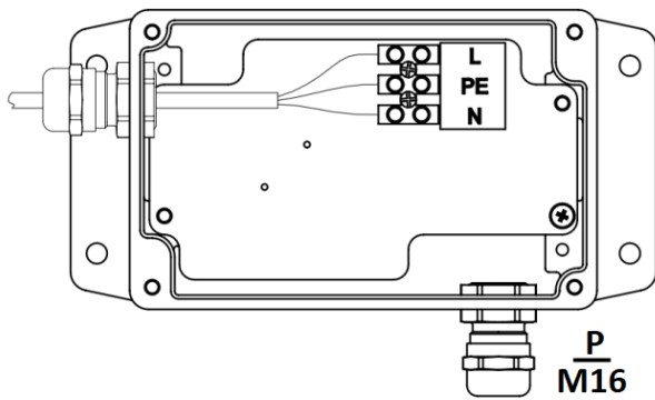
Вводная коробка
