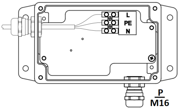
Вводная коробка
