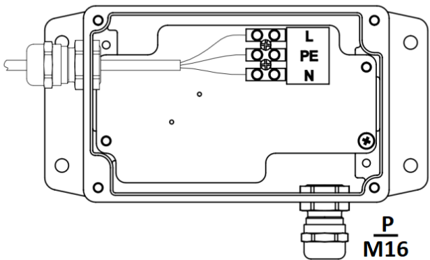
Вводная коробка
