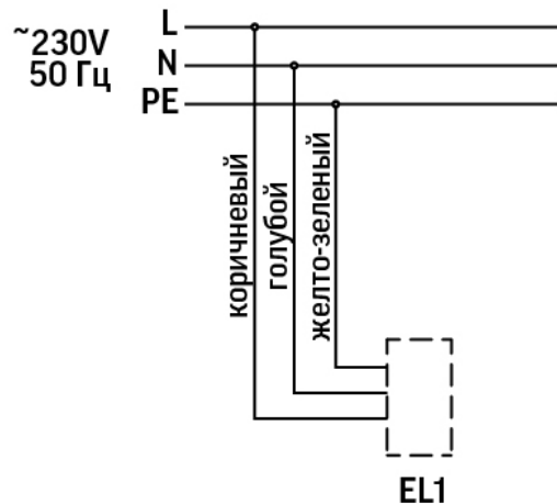
Рис.1 Встраиваемый
