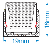
Алюминиевый профиль V4-NS-00.0047.STR-0003
