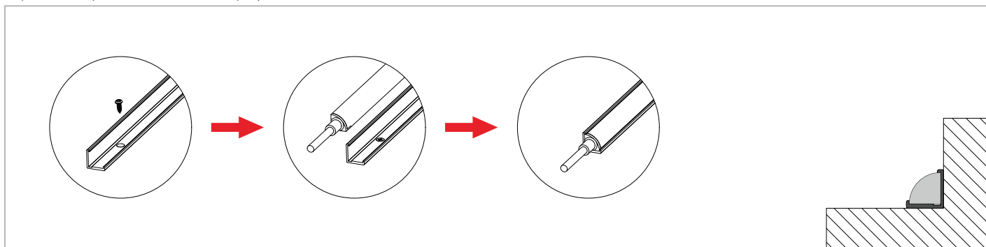
Вариант 4. Крепление на алюм. профиль
