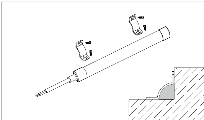
Вариант 3. Крепление на скобы
