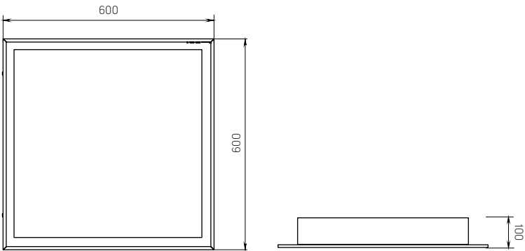
Габаритный чертёж
