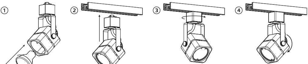
Рис. 1. Порядок монтажа
