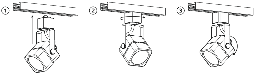
Рис. 1. Порядок монтажа
