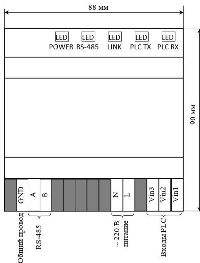
Рисунок 1. Чертеж корпуса Контроллер управления освещением AWADA SL-PLC
